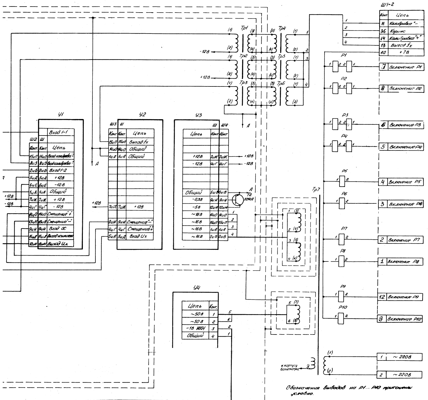
Вольтметр универсальный В7-21 БЛОК ИЗМЕРИТЕЛЬНЫЙ Схема электрическая принципиальная И25.171.41333
